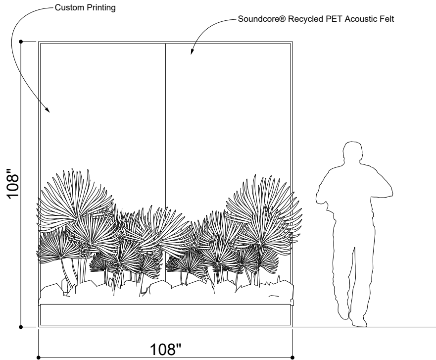
① ELEVATION 1
